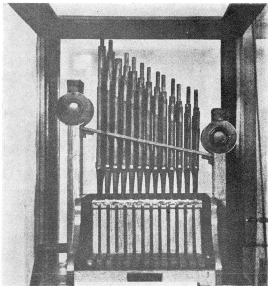
Figura 8. Reconstrucción del hydraulis de Aquinum.
