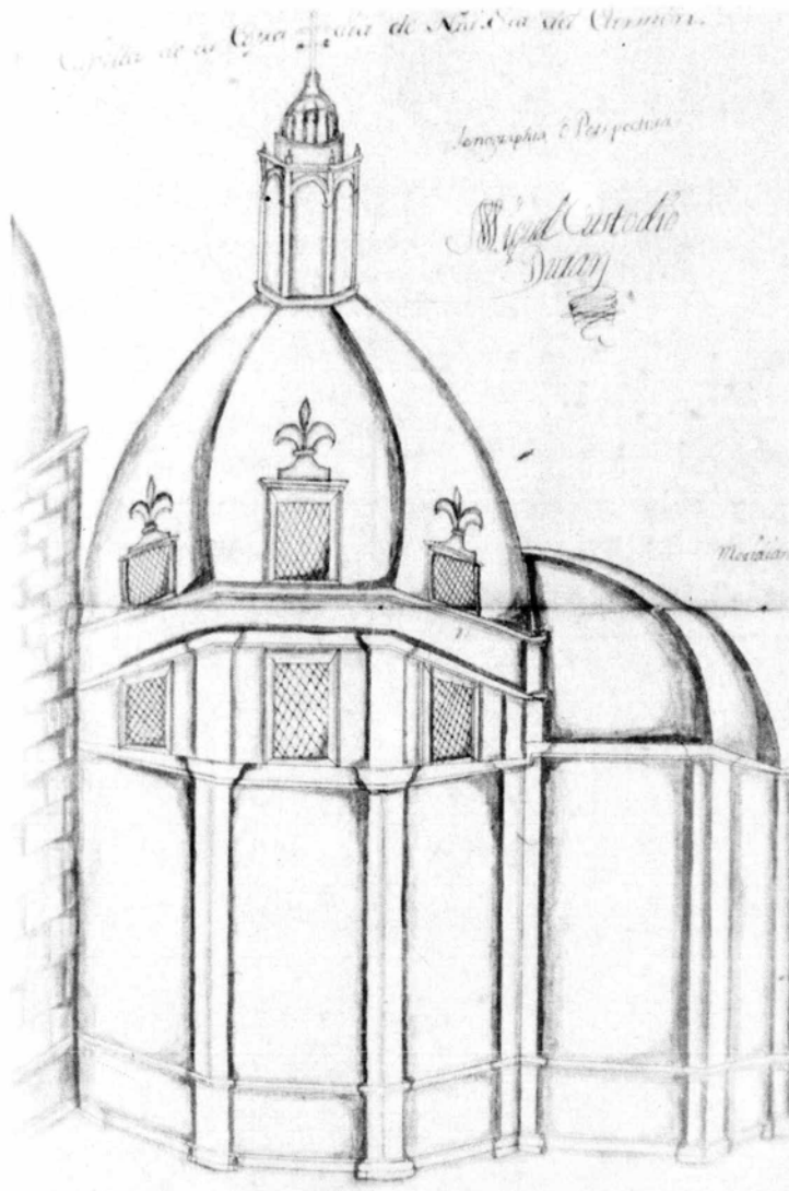
1. Alzado del exterior de la capilla de Nuestra Señora del Carmen en la iglesia de San Sebastián. Obra de Miguel Custodio Durán. Ciudad de México.
